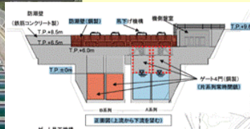
防潮ゲート 【取水口側】
