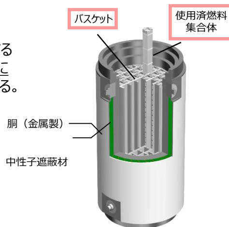
金属キャスク
