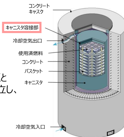
コンクリートキャスク
