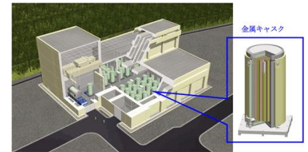
第2図 使用済燃料乾式貯蔵施設イメージ図 使用済燃料乾式貯蔵施設イメージ図
