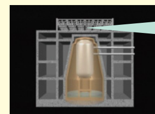
原子炉建屋の屋根を支えるトラス(イメージ)
