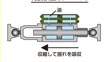
制震装置の取り付け
