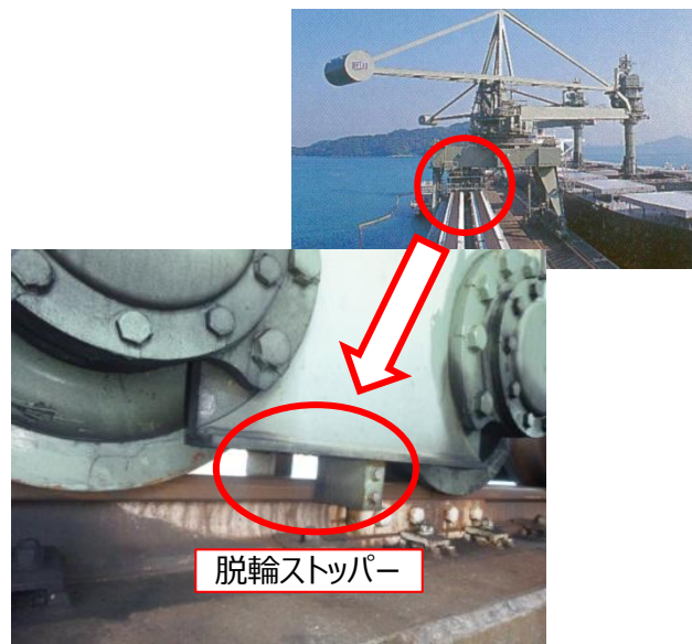
揚炭機の脱輪防止
