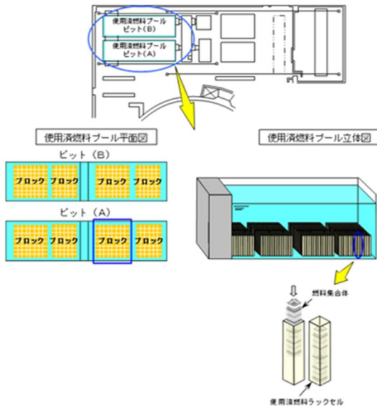
【使用済燃料貯蔵設備貯蔵能力増強概要図】
