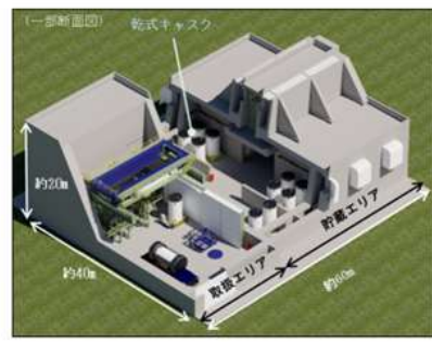
図1 乾式貯蔵建屋の全体鳥観図
