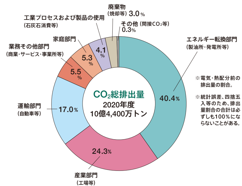
日本の部門別CO 2 排出量構成比(2020年度)
