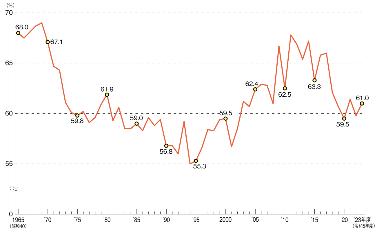
●年負荷率(送電端)の推移
