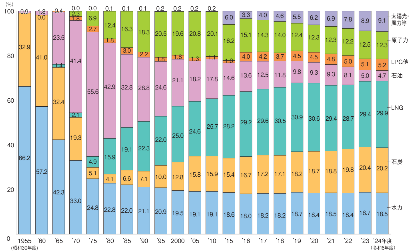
● 電源別発電設備構成比
