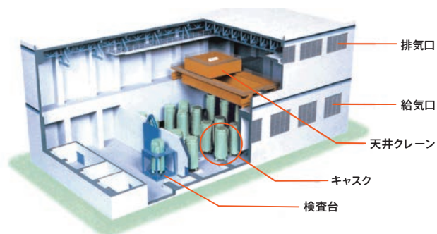
乾式キャスク貯蔵設備
