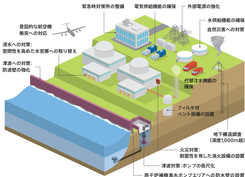
例：中部電力株式会社 浜岡原子力発電所 防波壁
