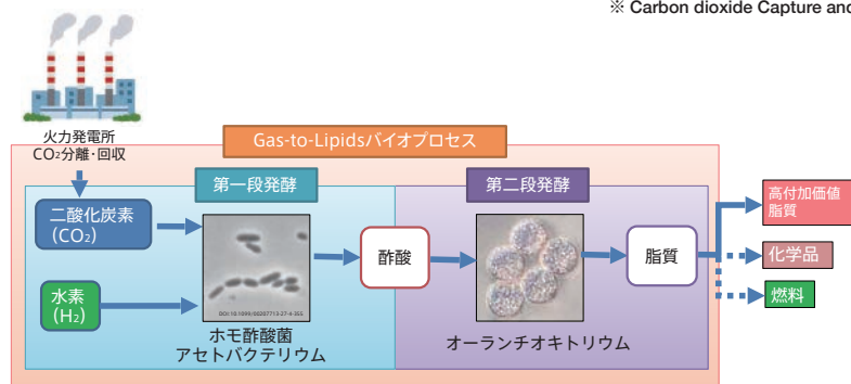
微生物を用いたCO 2 固定化技術
