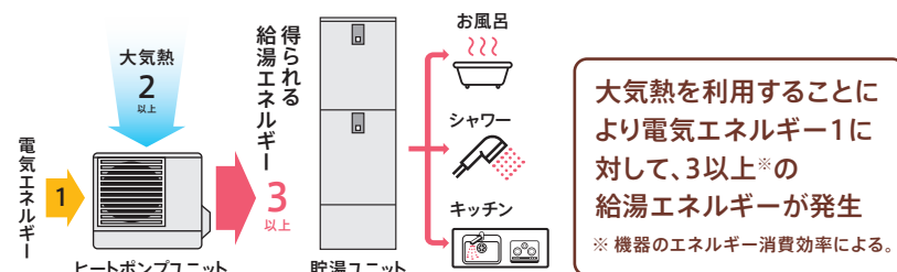
エコキュートの給湯システム概要図
