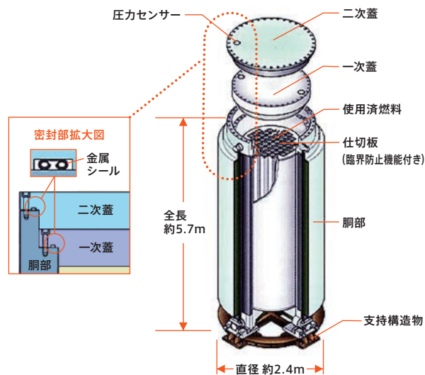
乾式キャスク
