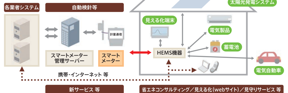
スマートメーター導入イメージ図
