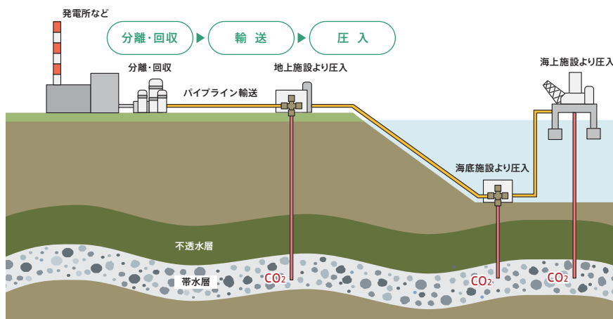
CO 2 地中貯留のイメージ
